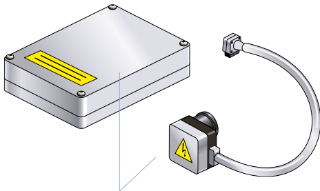
Elektronikus előtét és nagyfeszültségű indítószervezet
