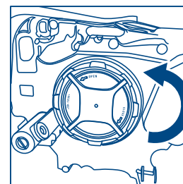
1 Vegye le a fényszóró fedelét.
