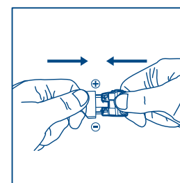
4 Dugja rá az izzóra a gépkocsi csatlakozóját (H1-es és H3-as típusoknál ügyelve a polarításra).
