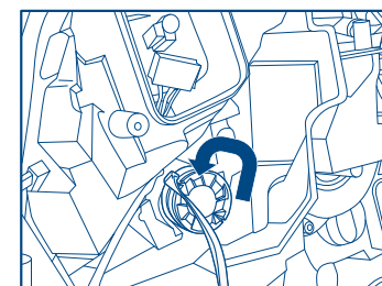
3 Vegye ki a központosító gyűrűt, és szerelje be a tartóba. Rögzítse a gyűrűt a fém kapoccsal. Szerelje be az izzót a tartóba. Enyhén elcsavarva rögzítse a helyén az izzót.
